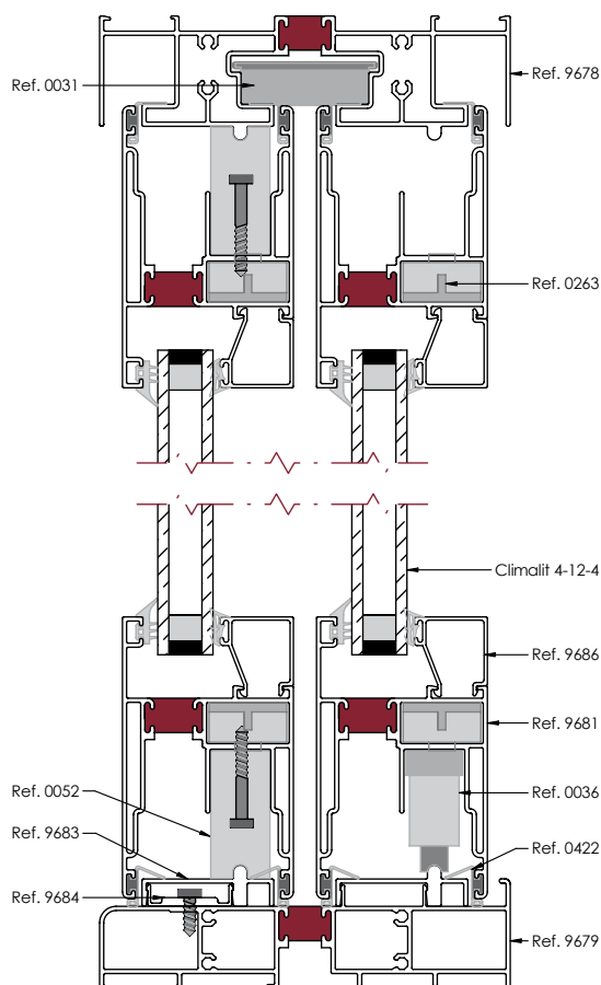
SECCIÓN VERTICAL
